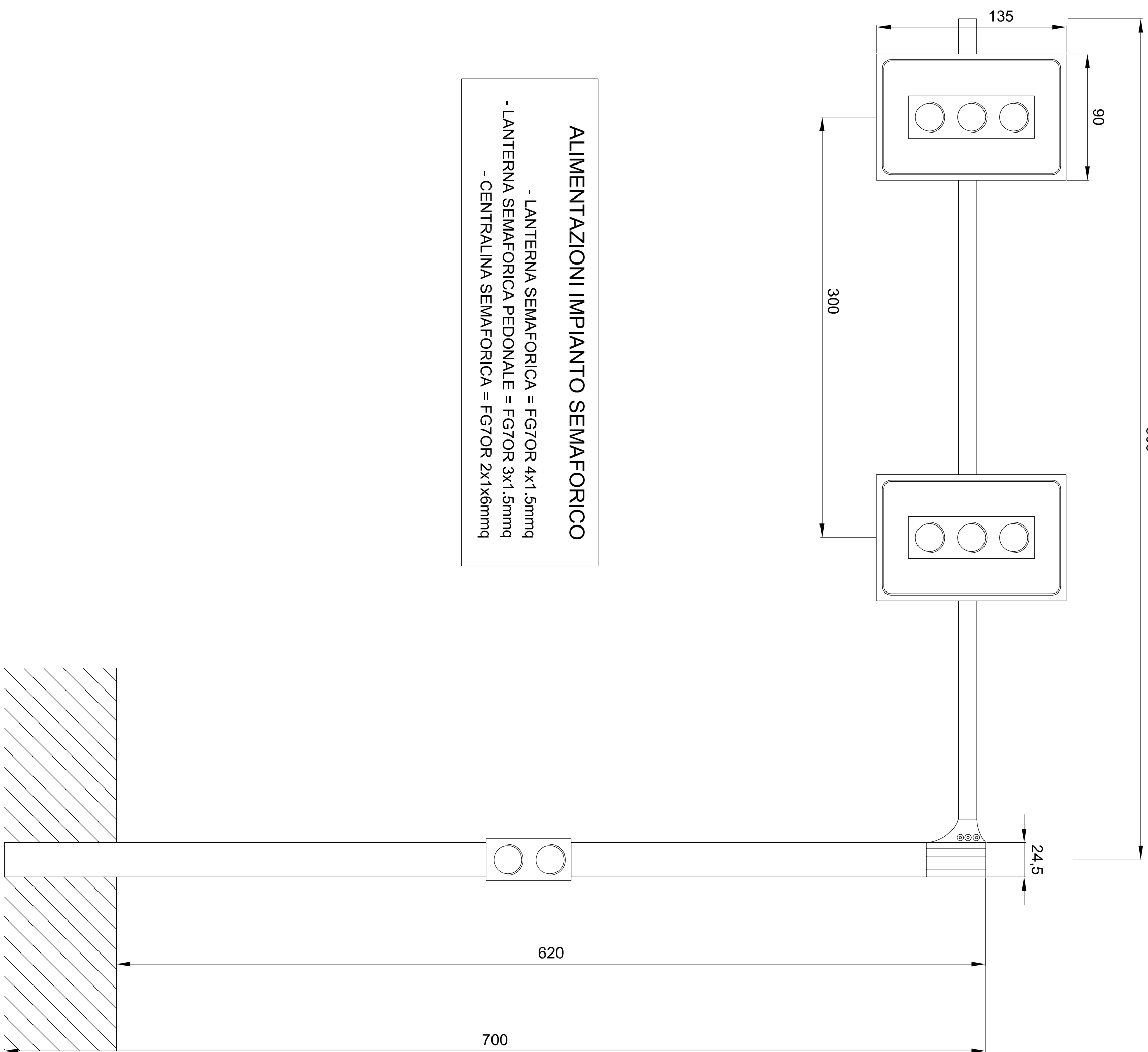
PARTICOLARE PALO SEMAFORICO
