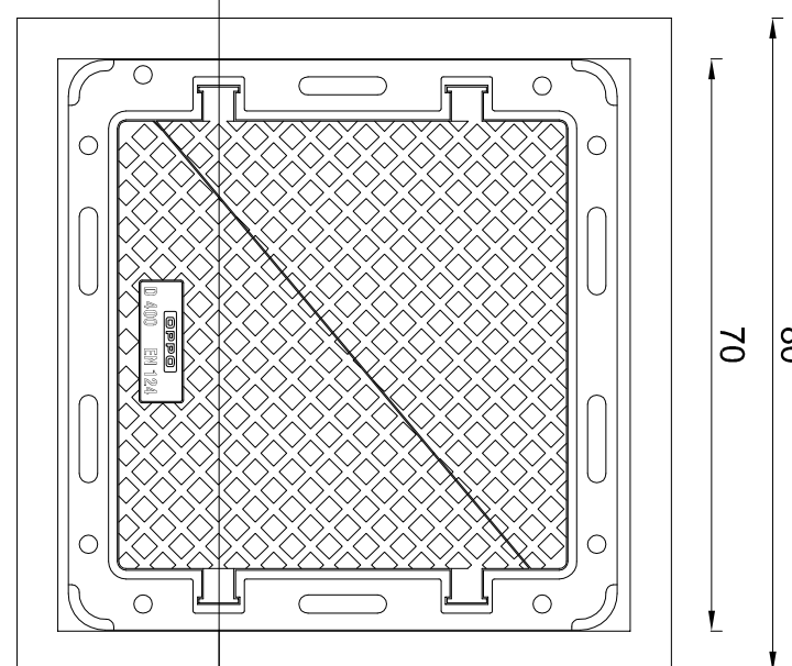
PIANTA POZZETTO I.P.
