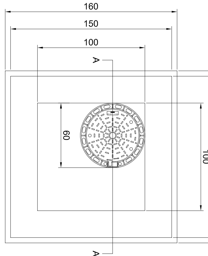
PIANTA POZZETTO B.T.
